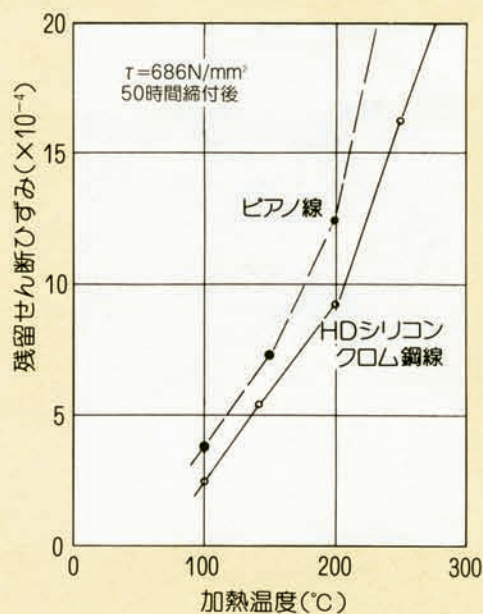
HDシリコンクロム鋼線の耐へたり性能
